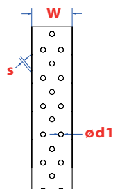
Bande perforée droite Windrispenband recht
