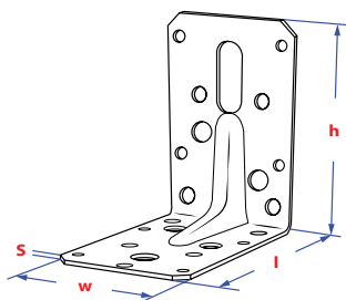
Equerre ajustable renforcée Winkelverbinder abstelbar mit Sicke
