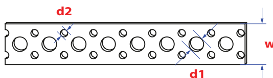
Bande perforée droite Windrispenband recht
