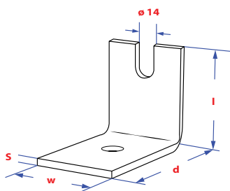
Equerre de fixation béton Betonwinkel
