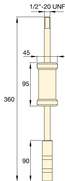
Afmetingen slaghamer (mm)
